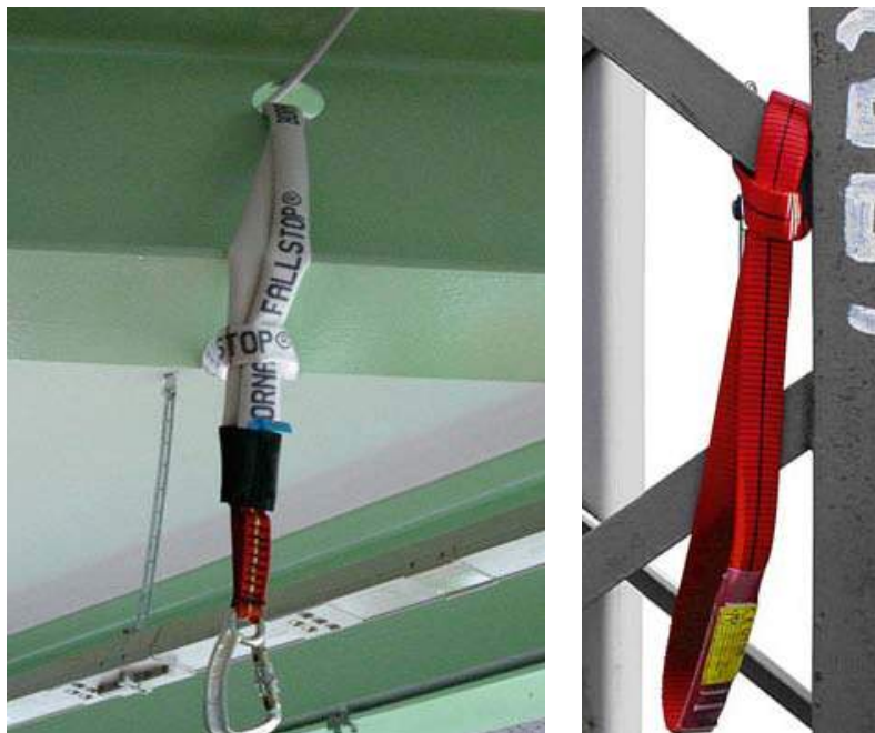
Bild 33: Beispiele für die Verwendung einer Bandschlinge als Anschlaghilfe
